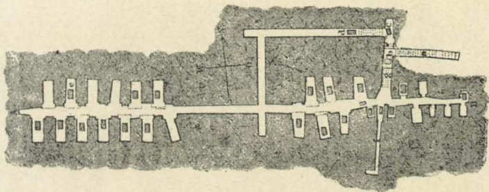
Fig. a LXX—Planta do Serapéum de Sakkárah. A galeria ao N. da entrada (a) era de serviço. Em (d) vê-se um sarcophago de granito, cuja tampa está em (c). Era conduzido para um dos nichos do fundo, ainda vazios. As galerias tem 350,0 metros d'extensão e 3,0 de largo por 5,50 d'alto.
