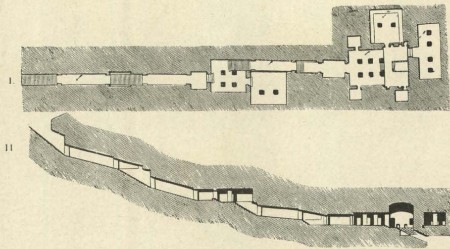
Fig. o LVI—Planta e corte longitudinal do hypogéo de Sethos I.
